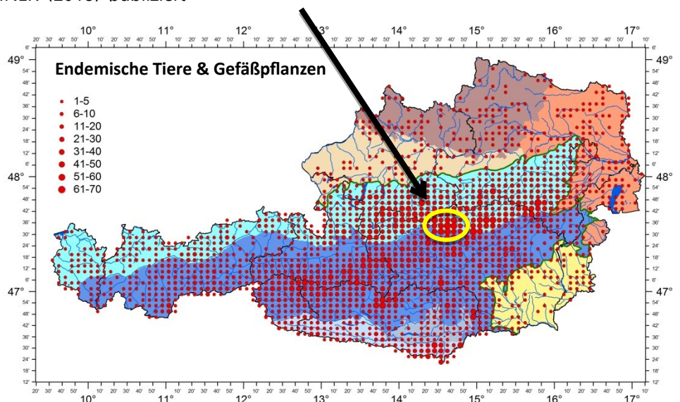
Karte aus RABITSCH & ESSL 2009 (Anzahl endemischer Arten in einem Rasterfeld (35 km 2 ))
